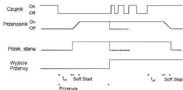
Sterowanie (1 czujnik)
