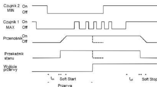
MIN / MAX sterowanie (2 czujniki)
